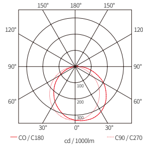
FNN1 27K-C90-1M 48.3lm/W 372lm
