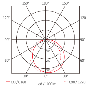
FNN1 40K-C90-1M 48.8lm/W 375.9lm
